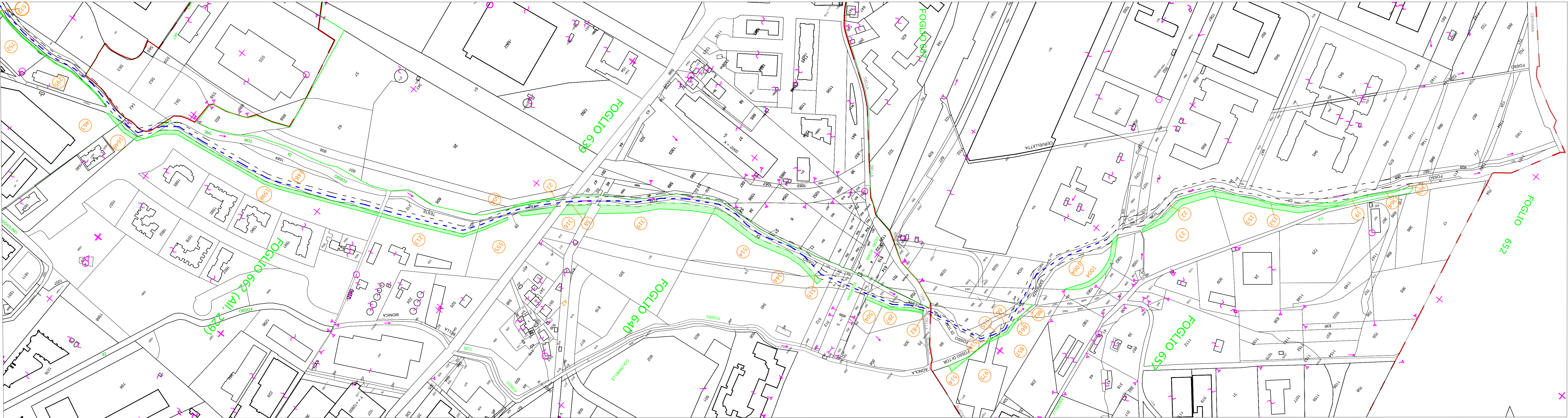
PLANIMETRIA STATO DI PROGETTO SU ESTRATTO DI MAPPA CATASTALE - Scala 1:2.000 - DA PROGRESSIVA 2+000 A PR. 3+800
